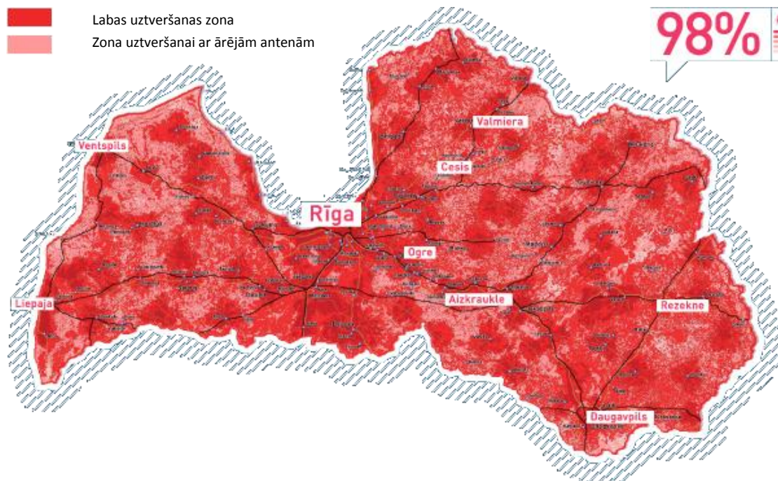
23. attēls. SIA TRIATEL bezvadu interneta pārklājums
